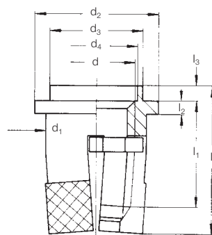
Type 0232 EXPANSIONERT 1 clinch
